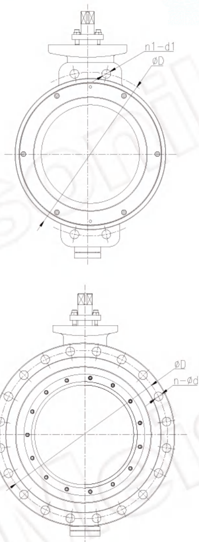
600LB阀体端面法兰连接尺寸
