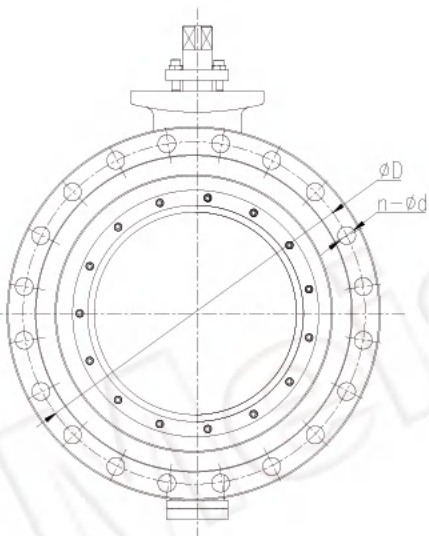
600LB阀体端面法兰连接尺寸
