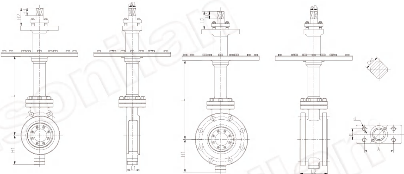
阀体结构尺寸
