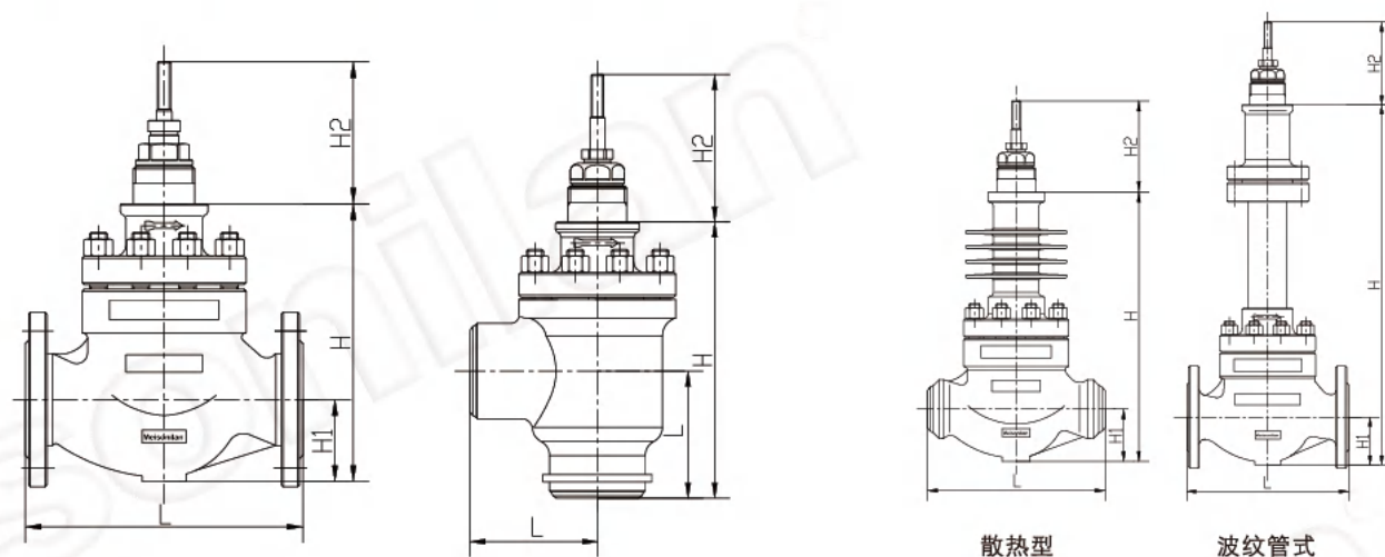
阀体结构尺寸
