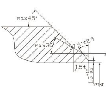
a. 管道壁厚 t \leq 22\text{mm} 的焊接端
